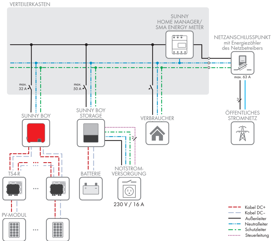
Abbildung 3: Verschaltungsübersicht (Beispiel)
